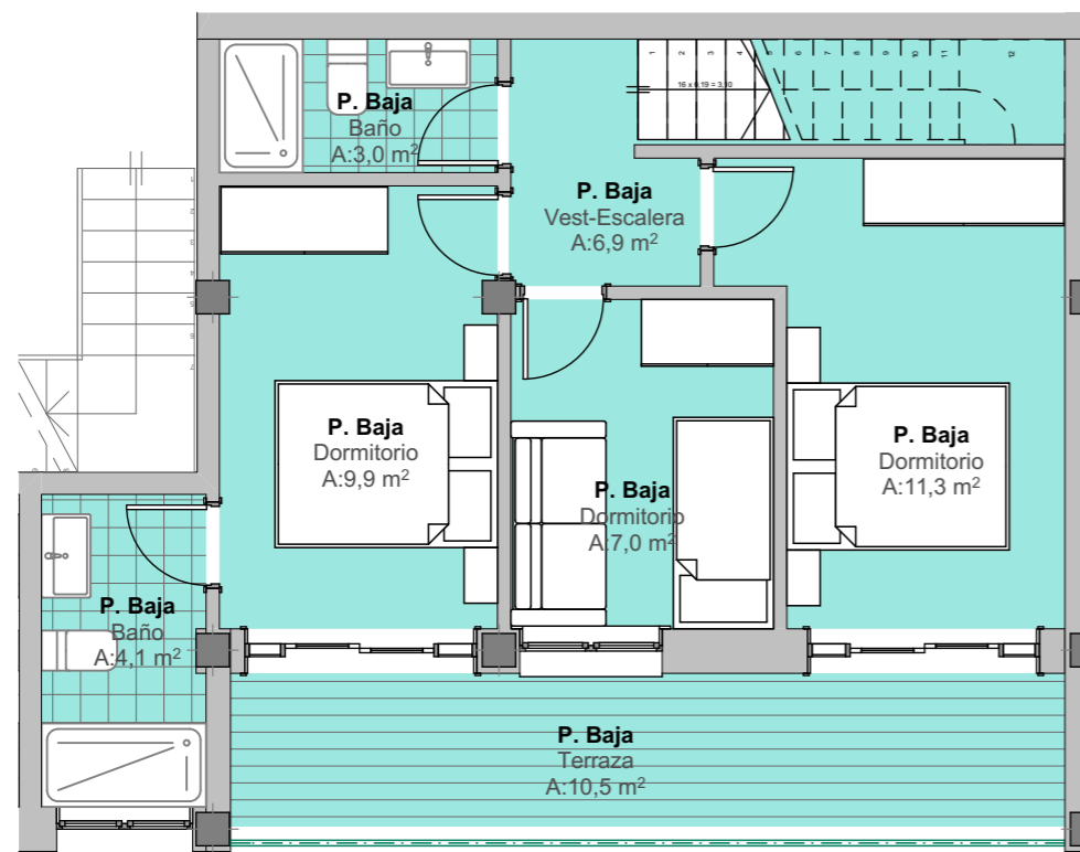
PLANTA TERCERA
