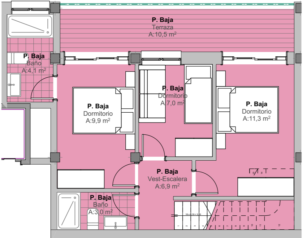
PLANTA TERCERA
