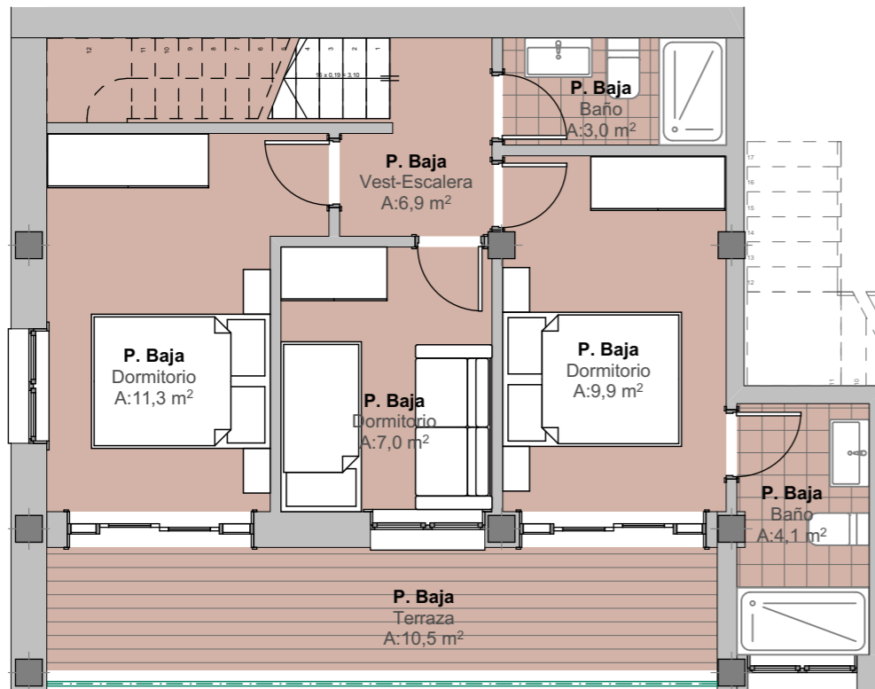
PLANTA TERCERA
