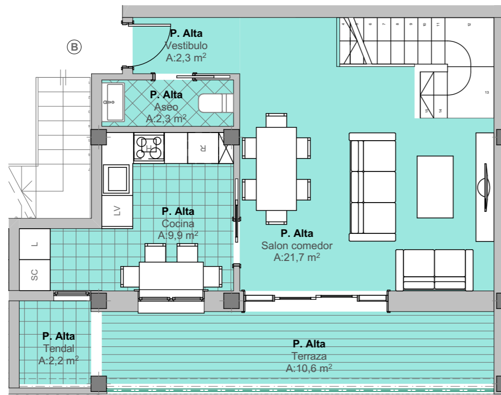
PLANTA ATICO
