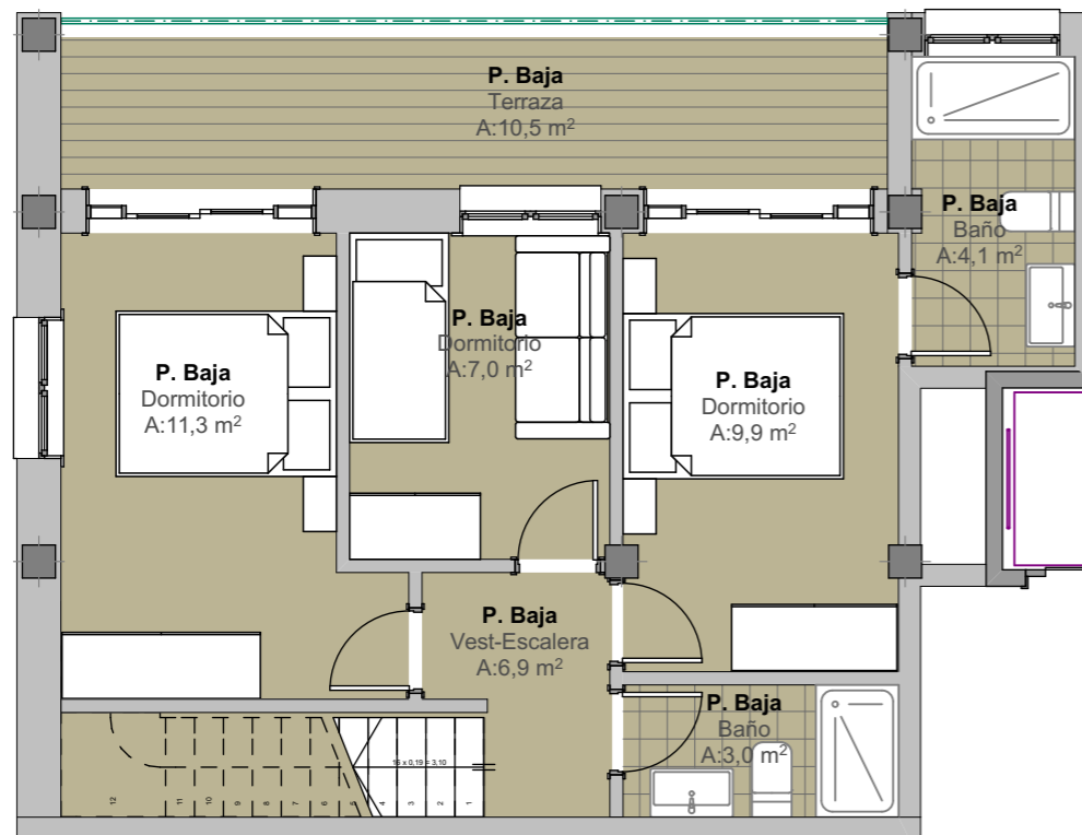
PLANTA TERCERA
