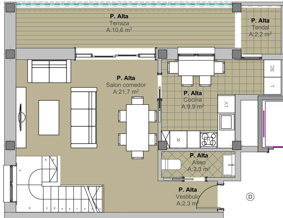
PLANTA ATICO
