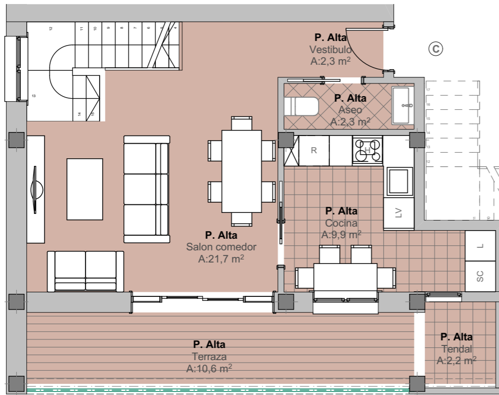
PLANTA ATICO
